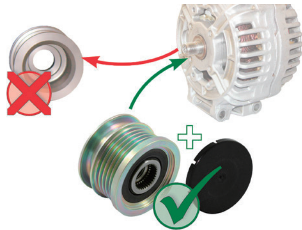
画像 1： オーバーランニングオルタネータープーリーの高剛性ベルトプーリーの変更
